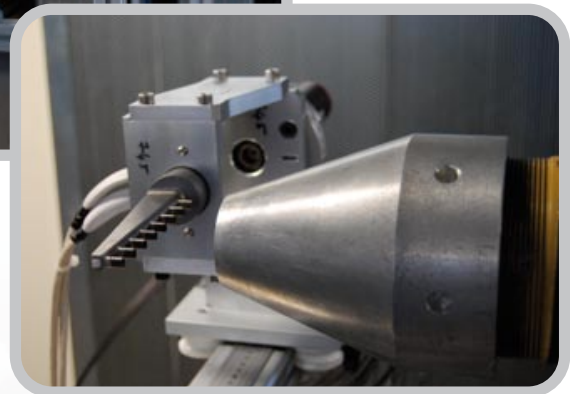
🔗 Etalonnage d'un peigne de mesures pour performances moteur / Calibration for a probes used for engine performance determination
